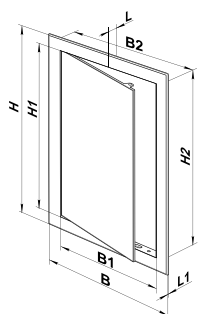
Пластиковые ревизионные дверцы двухстороннего монтажа с поверхностью для покраски
